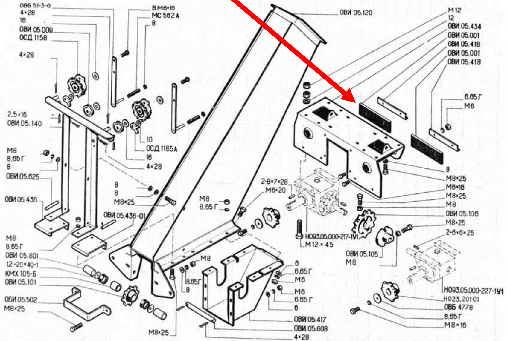
Рис. 25. Секция нижняя ОВИ 05.110.
